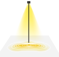
AB4 - 145°x 60° η 83,9% - G*3
